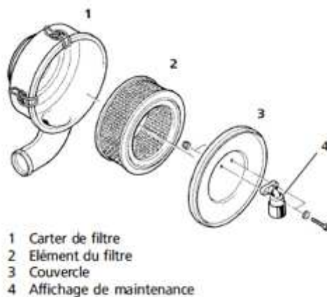
Fig. 12 Filtre d'aspiration, IK150, IK18.1, IK180
