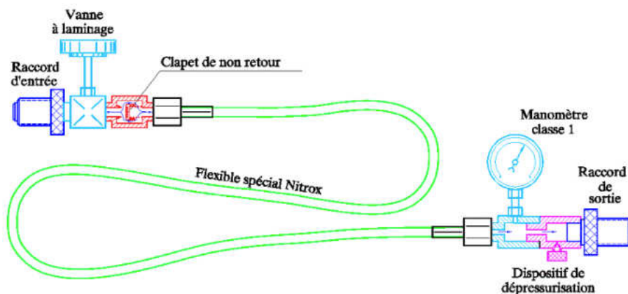
Schéma d'Henri Le Bris (Ref.3)
